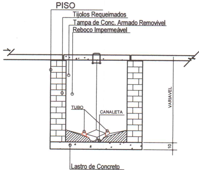
2 Corte CI Obs.: As cotas prevalecem no desenho. Esc.: S/ Escala
