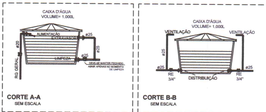
PLANTA BAIXA CAIXA D'ÁGUA (1000L) SEM ESCALA
